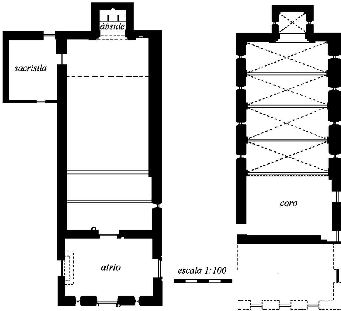
Planta baja
